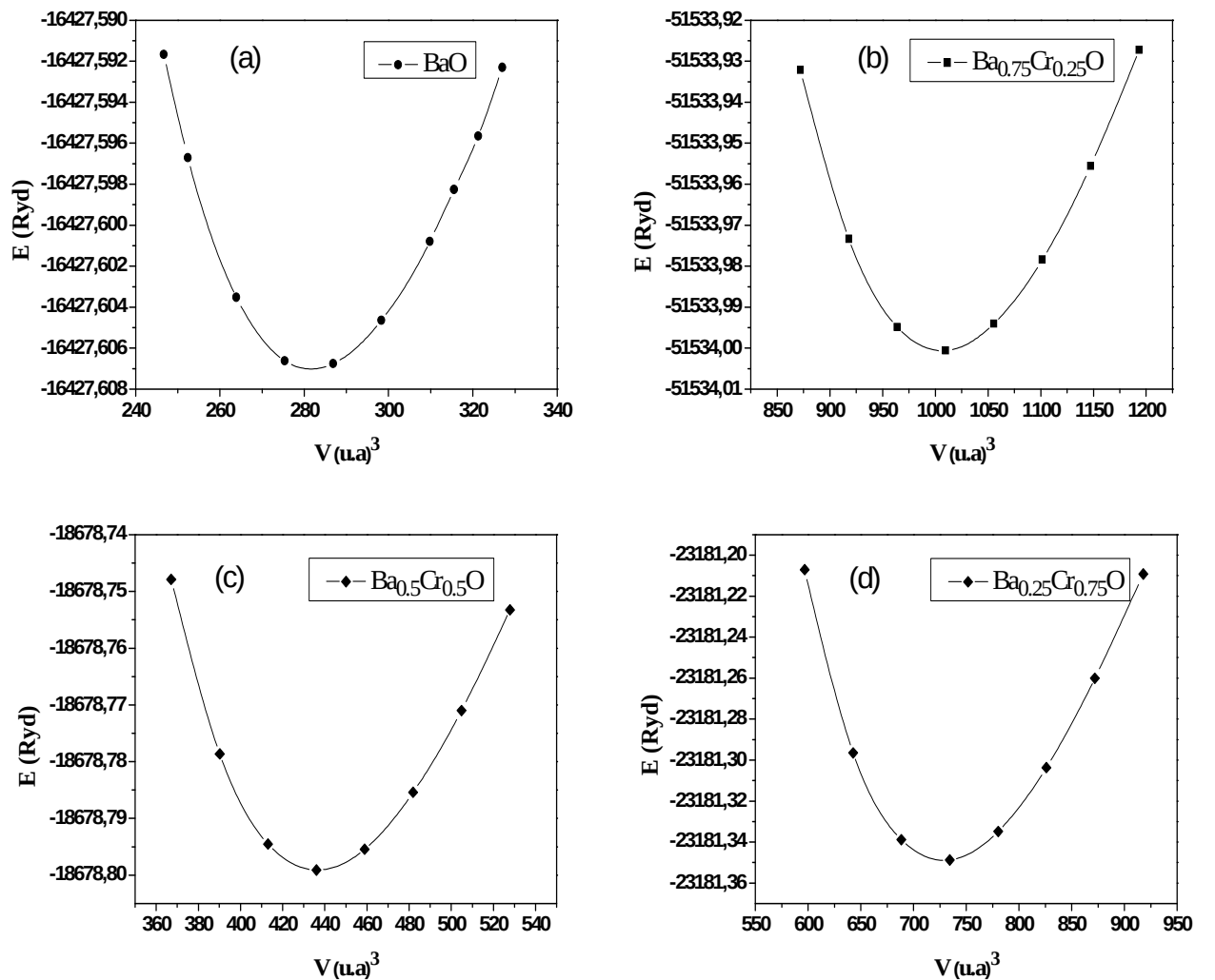
Figure III.1 : Variations des énergies totales en fonction des volumes des matériaux \text{BaO} et \text{Ba}_{1-x}\text{Cr}_x\text{O} . (a) \text{BaO} , (b) \text{Ba}_{0.75}\text{Cr}_{0.25}\text{O} , (c) \text{Ba}_{0.5}\text{Cr}_{0.5}\text{O} et (d) \text{Ba}_{0.25}\text{Cr}_{0.75}\text{O} .
