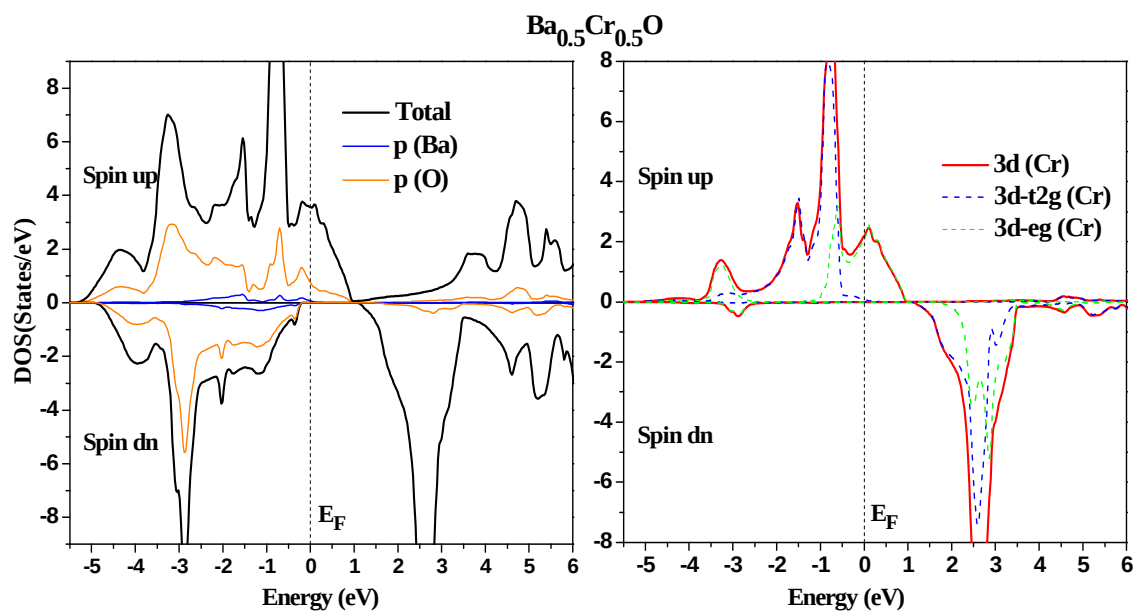
Figure III-4 : Les DOS totales et partielles des spins majoritaires ( up ) et spins minoritaires ( dn ) de \text{Ba}_{0.5}\text{Cr}_{0.5}\text{O} .
