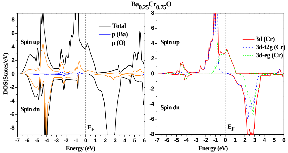
Figure III-5 : Les DOS totales et partielles des spins majoritaires ( up ) et spins minoritaires ( dn ) de \text{Ba}_{0.25}\text{Cr}_{0.75}\text{O} .
