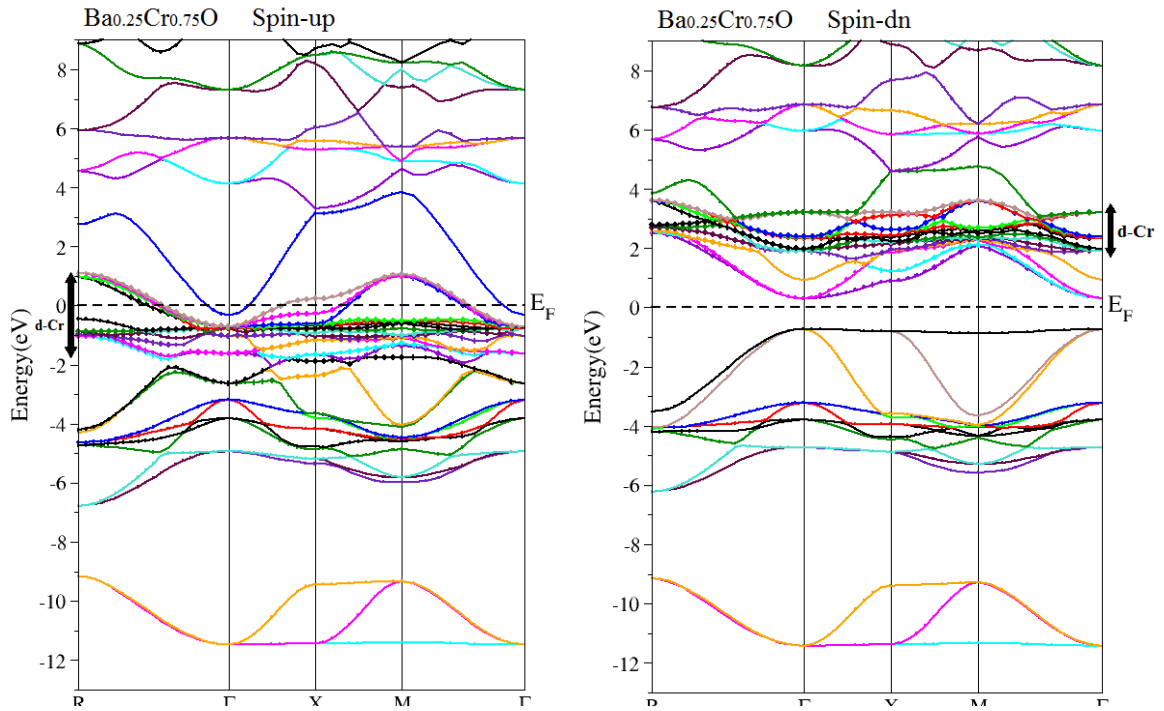
Figure III.9 : Les structures de bandes des spins majoritaires ( up ) et spins minoritaires ( dn ) de \text{Ba}_{0.25}\text{Cr}_{0.75}\text{O} .
