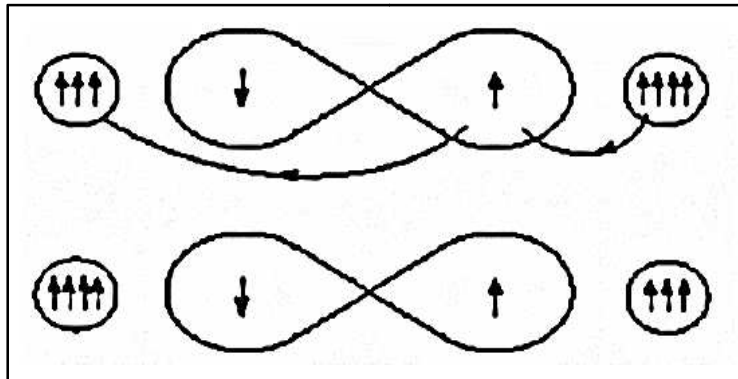
Figure I-2 : Double échange : cas de deux ions \text{Mn}^{4+} et \text{Mn}^{3+} séparés par un ion oxygène. Au même moment où un électron de l'ion \text{Mn}^{4+} saute vers l'oxygène, celui-ci cède un électron vers l'autre ion \text{Mn}^{3+} . Ceci n'est possible que si les deux ions de Mn possèdent des spins parallèles.
